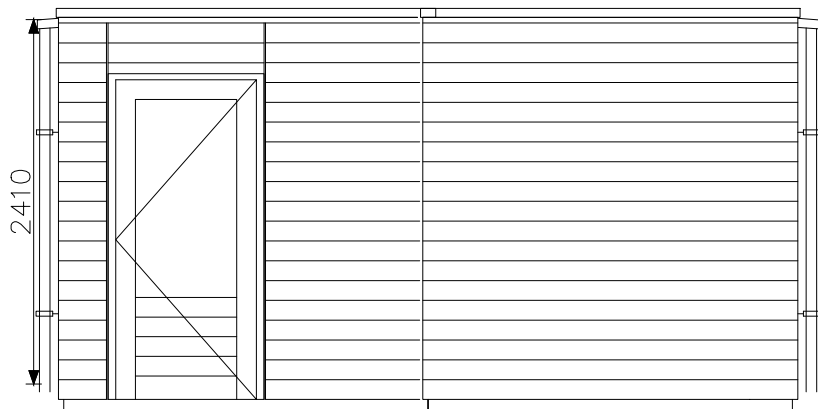
zijgevel Rechts
