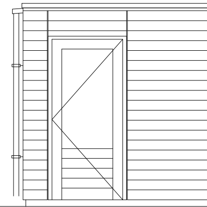
zijgevel Rechts
