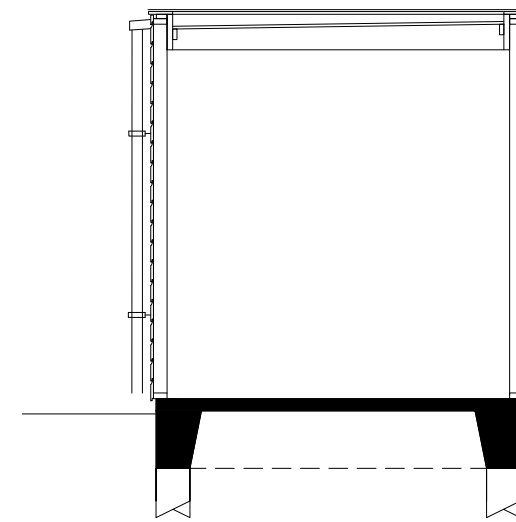
doorsnede "op palen"
